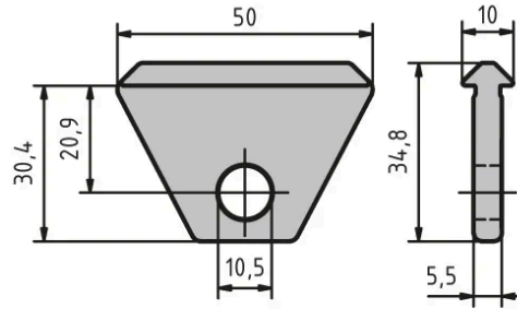
Nut 6
