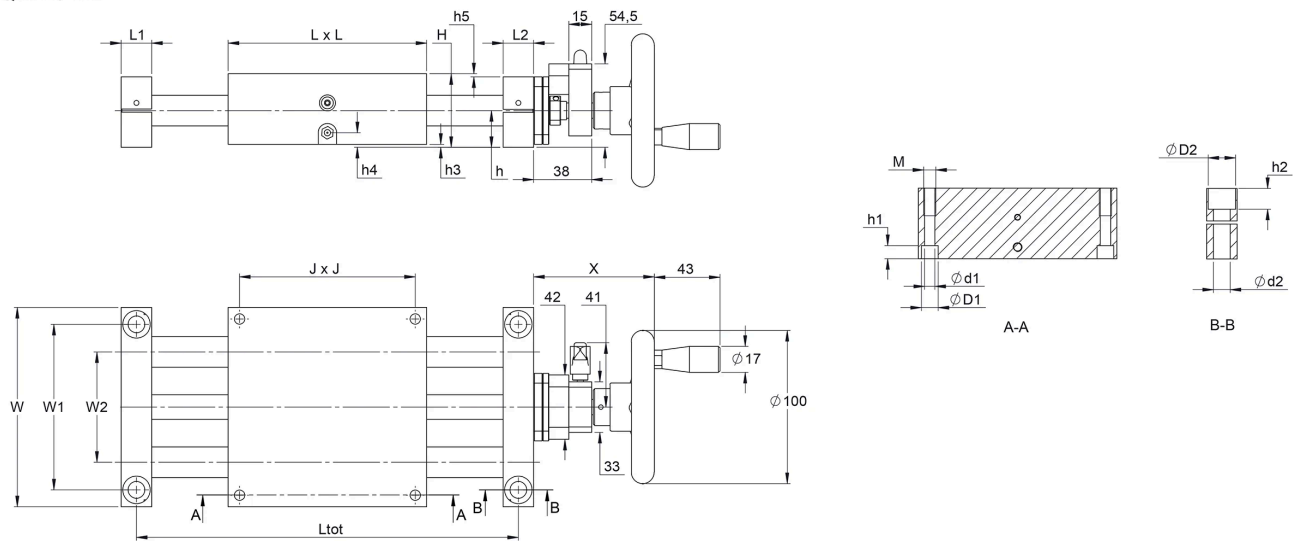
QME20-WL
